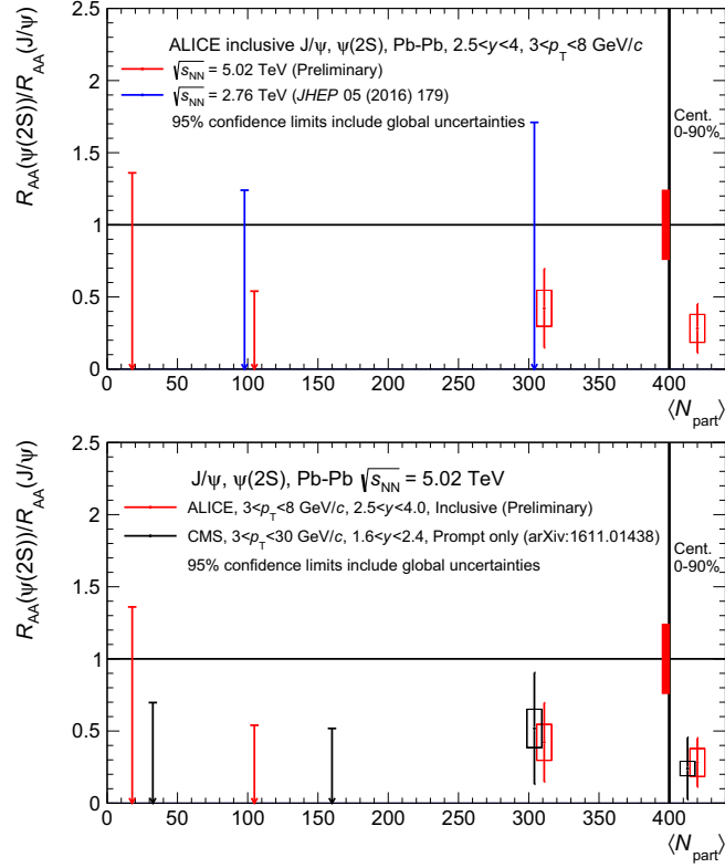
FIGURE 7: Double-rapport R_{AA}^{\psi(2S)}/R_{AA}^{J/\psi} en fonction de N_{\text{part}} comparé aux valeurs à \sqrt{s_{NN}} = 2.76 TeV (Haut) et aux valeurs de CMS à \sqrt{s_{NN}} = 5.02 TeV. Pour les intervalles où le signal ne peut pas être extrait, la limite à 95% de confiance est montrée. L'incertitude systématique globale est dessinée autour de l'unité. L'incertitude globale est incluse dans le calcul des intervalles de confiances. La valeur à N_{\text{part}} > 400 correspond à la valeur intégrée en centralité (0-90%).
