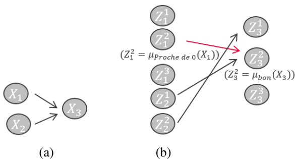
Figure 2 – Exemples fictifs de graphes causaux construits, avec les variables d'origine (a), avec les nouvelles variables (b)
