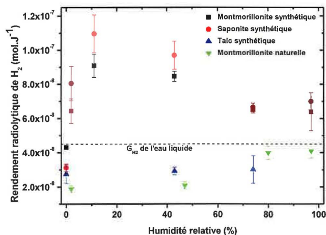
Figure 1. Rendements radiolytiques de production de dihydrogène mesurés pour différents matériaux argileux, à différentes humidités relatives.
